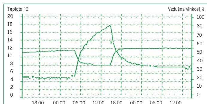
Obrázek 1: Časová závislost teploty a relativní vlhkosti v evangelickém kostele v Glarusu (Švýcarsko) Až do čtyř hodin do rána se teplota držela na 5 °C (křivka označena T), pak došlo k zapnutí otopné soustavy a teplota vystoupila až na 18 °C, v 15:00 bylo topení vypnuto a budova rychle vychladla na 8 °C. Do začátku topení byla relativní vlhkost kolem 55 %, během topení klesla až na 40 % a při následném ochlazení vystoupila k 60 %.
